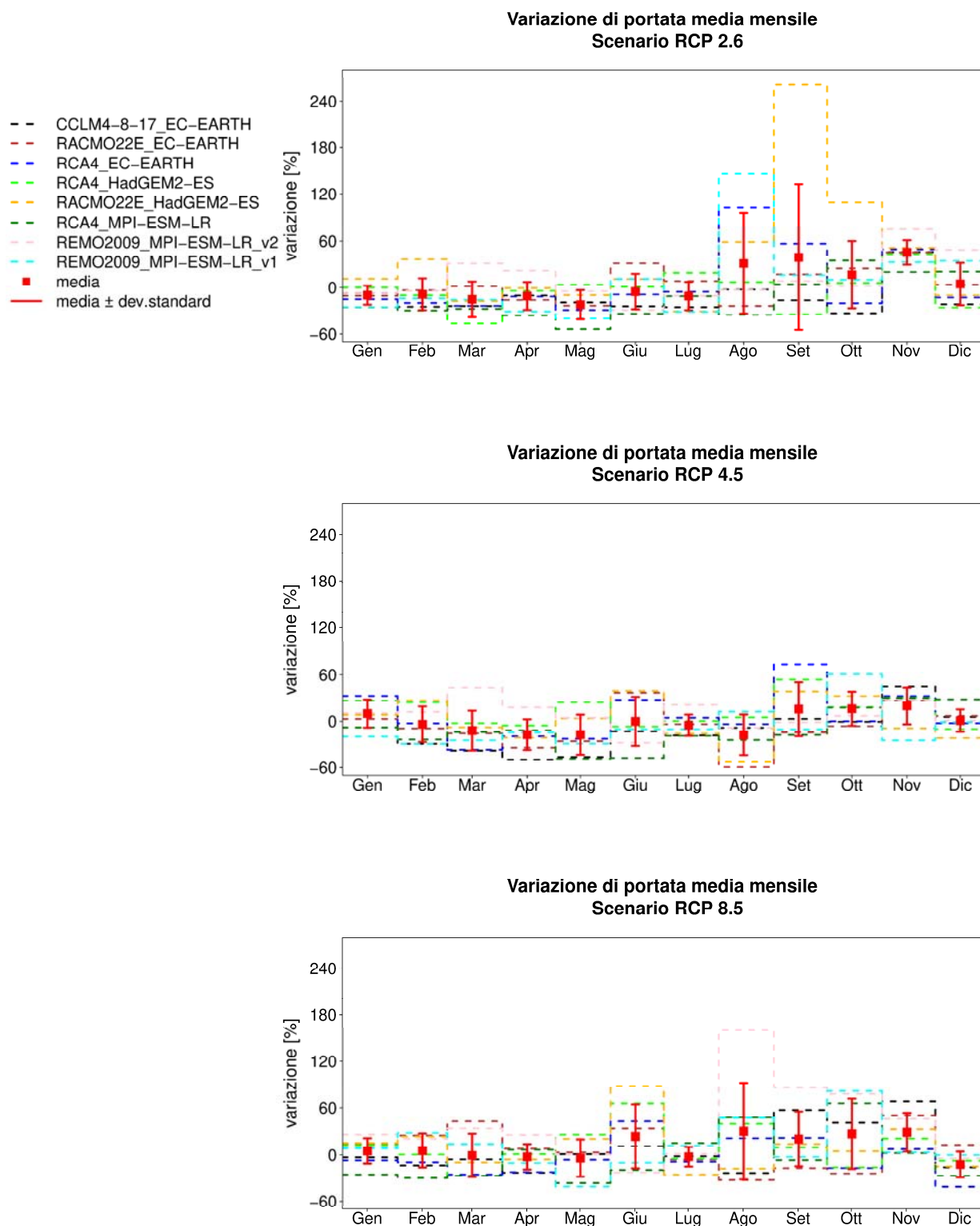
Figura A7. Variazioni di portata media mensile fornite dalle diverse catene modellistiche per il bacino Traversa Santa Venere, per i diversi scenari RCP. Sono indicate anche la media di ensemble e la deviazione standard della variazione.
