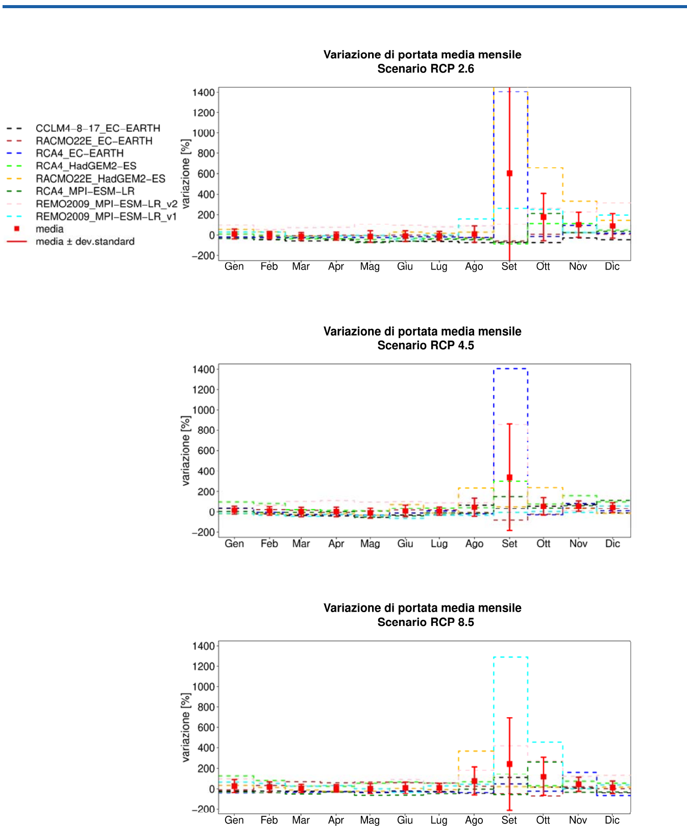
Figura A2. Variazioni di portata media mensile fornite dalle diverse catene modellistiche per il bacino Locone, per i diversi scenari RCP. Sono indicate anche la media di ensemble e la deviazione standard della variazione.
