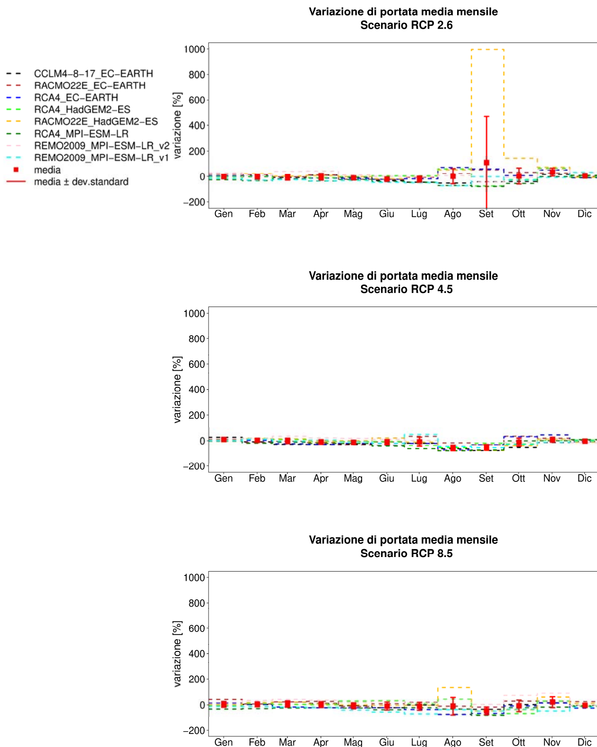
Figura A5. Variazioni di portata media mensile fornite dalle diverse catene modellistiche per il bacino Pertusillo, per i diversi scenari RCP. Sono indicate anche la media di ensemble e la deviazione standard della variazione.
