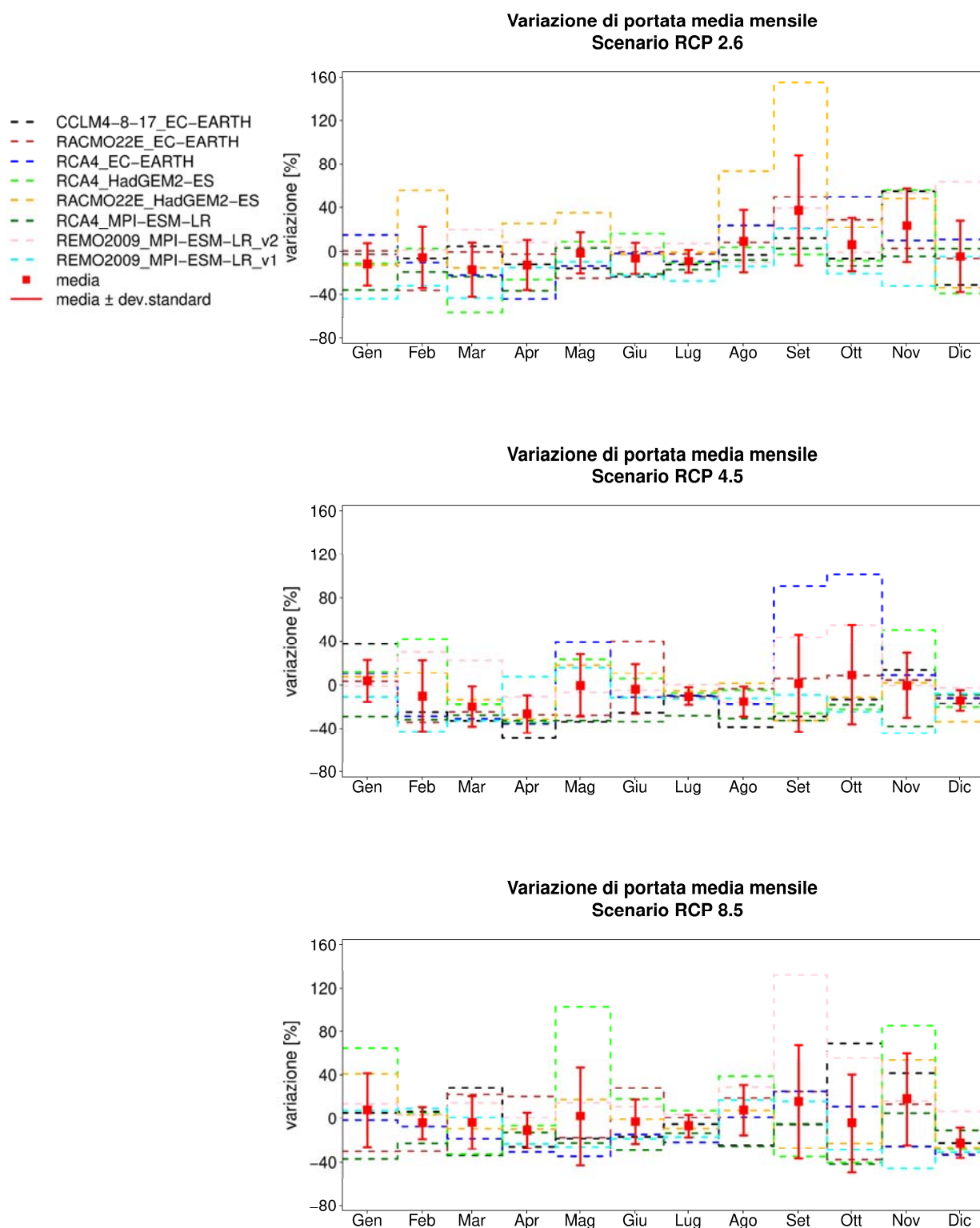
Figura A8. Variazioni di portata media mensile fornite dalle diverse catene modellistiche per il bacino Traversa Sarmento, per i diversi scenari RCP. Sono indicate anche la media di ensemble e la deviazione standard della variazione.
