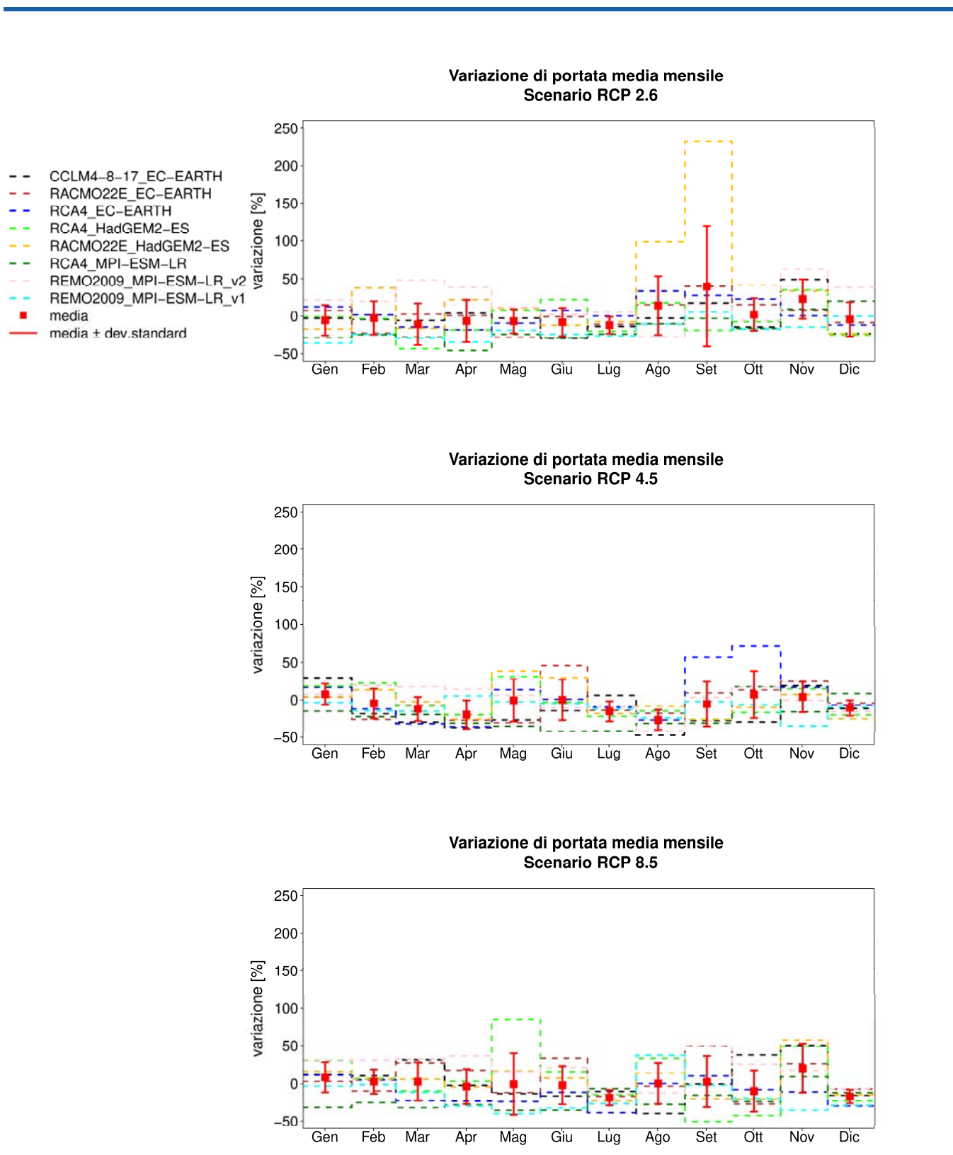
Figura A3. Variazioni di portata media mensile fornite dalle diverse catene modellistiche per il bacino Monte Cotugno, per i diversi scenari RCP. Sono indicate anche la media di ensemble e la deviazione standard della variazione.
