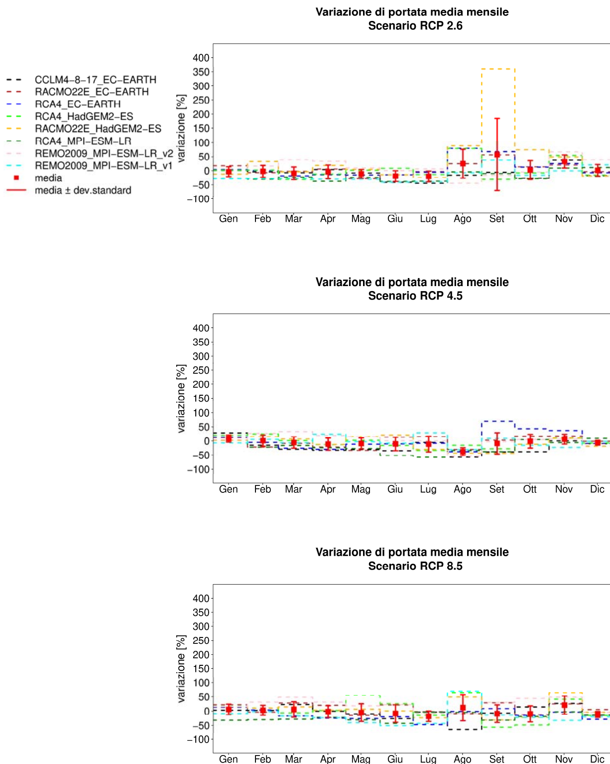
Figura A6. Variazioni di portata media mensile fornite dalle diverse catene modellistiche per il bacino Traversa Agri, per i diversi scenari RCP. Sono indicate anche la media di ensemble e la deviazione standard della variazione.
